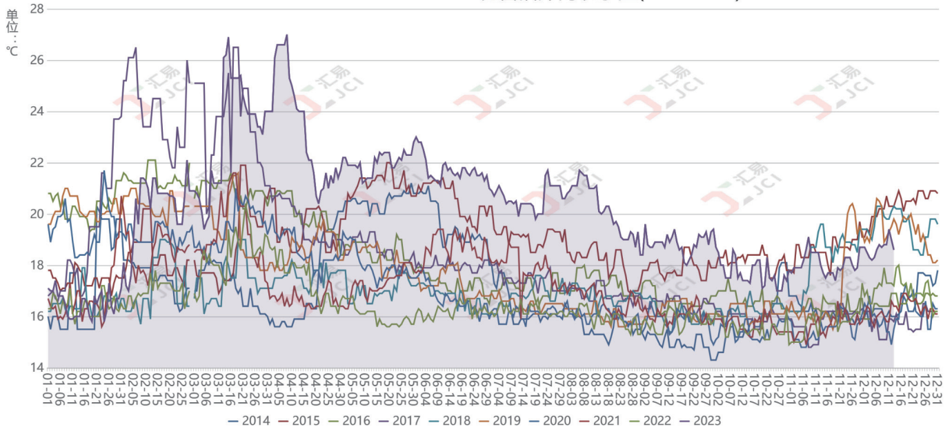
JCI: 2014-01-01~2023-12-15秘鲁沿岸海表水温('Chicama')
