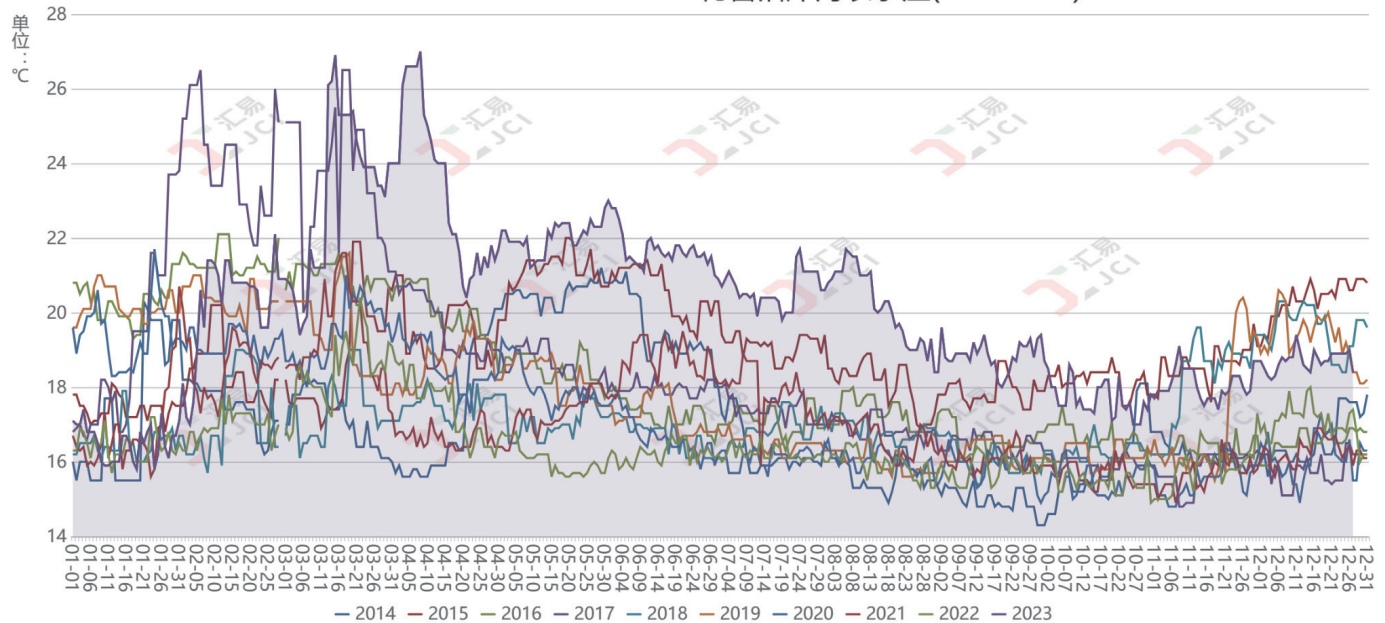
JCI: 2014-01-01~2023-12-29秘鲁沿岸海表水温('Chicama')
